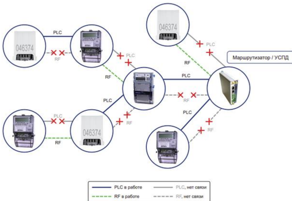
Рисунок 1.4 – Схема работы сети G3-PLC HYBRID PLC&RF
