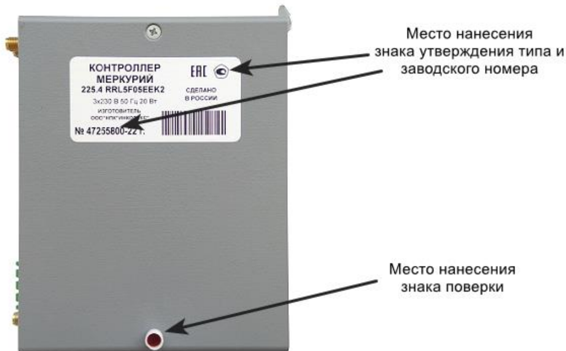
Рисунок 1.6 – Схема пломбирования
